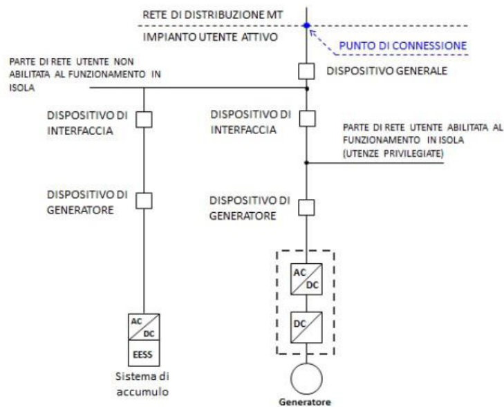
Fig.4-c: Sistema di accumulo posizionato nella parte di impianto in corrente alternata a monte del contatore dell'energia generata
