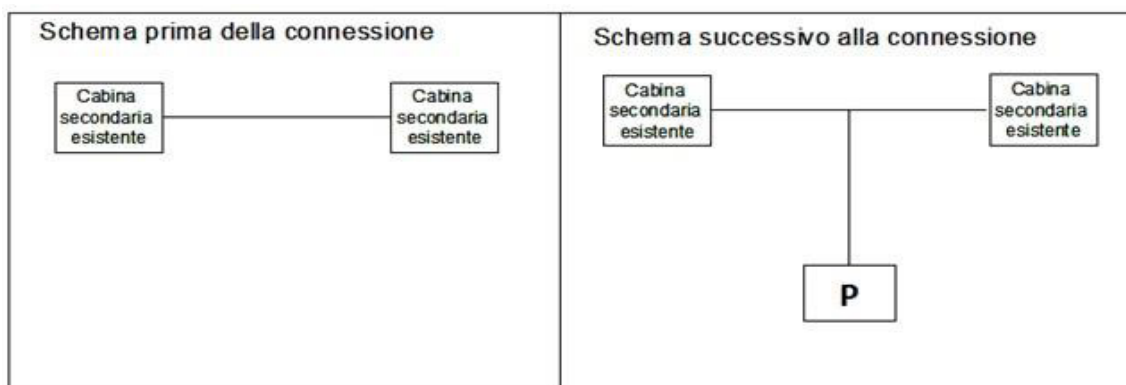
Figura 8- Inserimento in derivazione rigida a T su linea esistente
