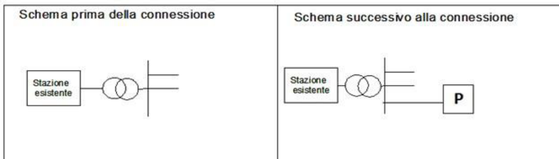
Figura 5- Inserimento in antenna da stazione AT/MT
